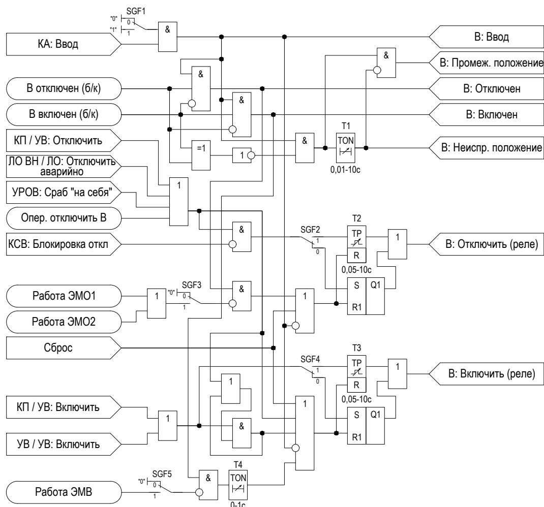
Рисунок 2.33 – Функциональная схема логики выключателя
