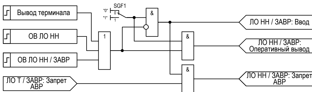
Рисунок 2.25 – Функциональная схема логики запрета АВР
